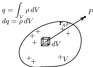
Volume charge (d)
